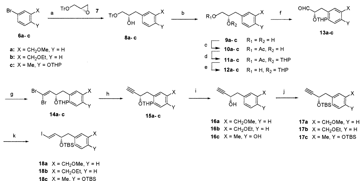
Scheme 2. Preparation of optically active vinyl iodide 18a–c . Reagents: (a) Mg, CuI, THF then 7 ; (b) AcOH, THF, H 2 O; (c) AcCl, 2,4,6-collidine, CH 2 Cl 2 ; (d) DHP, p -TsOHH 2 O, CH 2 Cl 2 ; (e) 2 N NaOH, MeOH; (f) (COCl) 2 , DMSO, Et 3 N, CH 2 Cl 2 ; (g) CBr 4 , Ph 3 P, Et 3 N, CH 2 Cl 2 ; (h) n -BuLi, THF; (i) 4 N HCl–dioxane, MeOH; (j) TBSCl, imidazol, DMF; (k) Cp 2 ZrClH, I 2 , THF.
